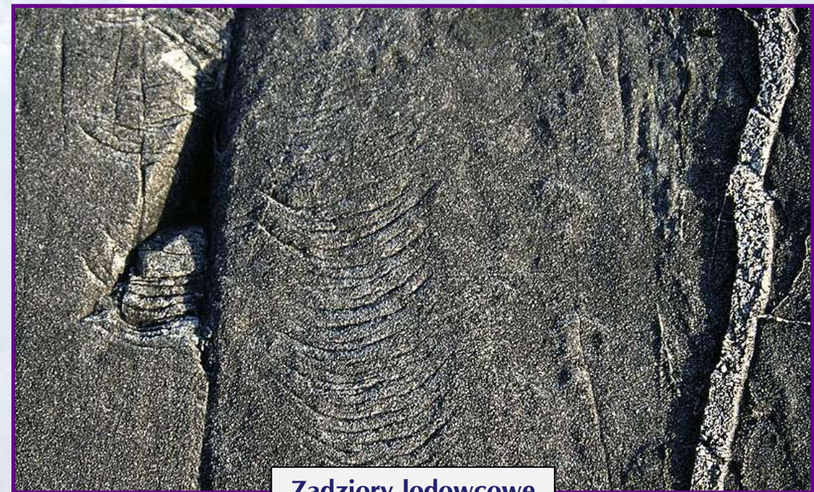
Zadziory lodowcowe
