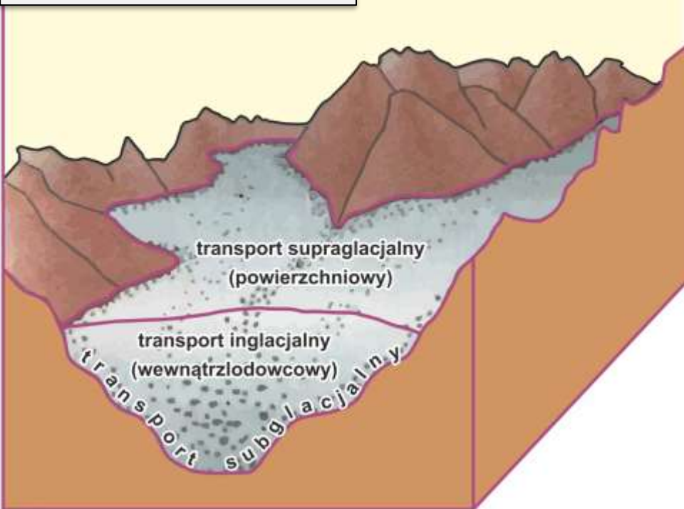
Materiał transportowany przez lodowiec górski
