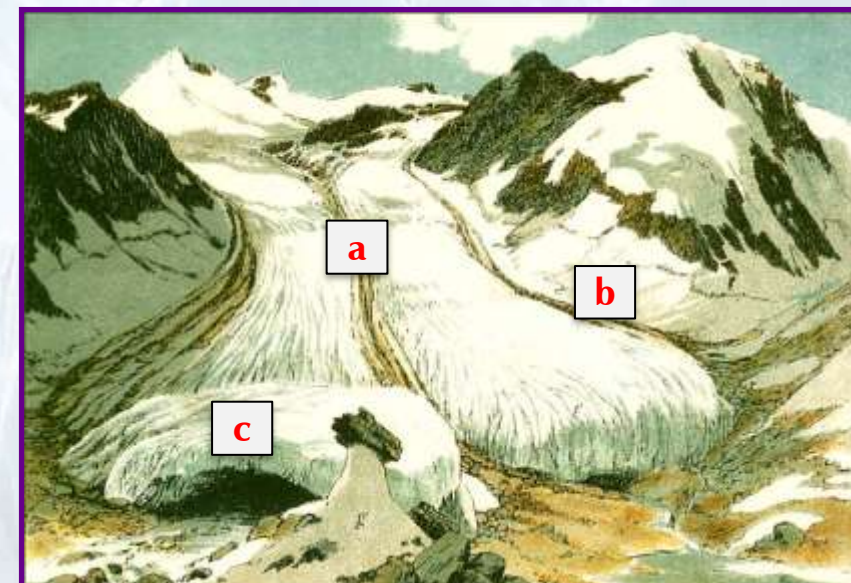
Lodowiec górski: a – morena środkowa, b – morena boczna, c – czoło lodowca, gdzie powstaje morena czołowa.
