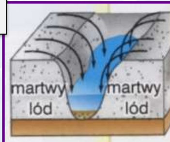
Powstawanie kemów
