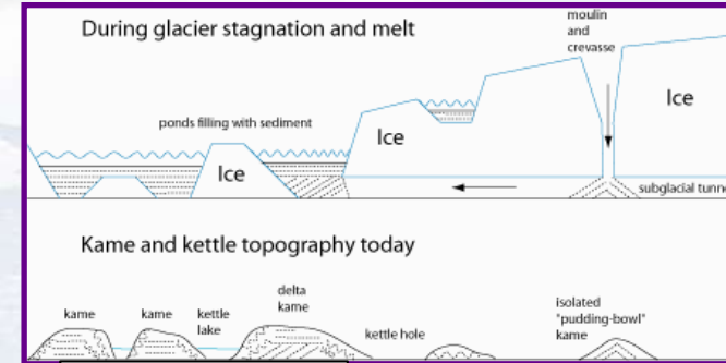
Powstawanie kemów
